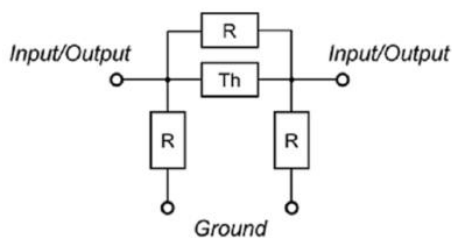
等価回路
